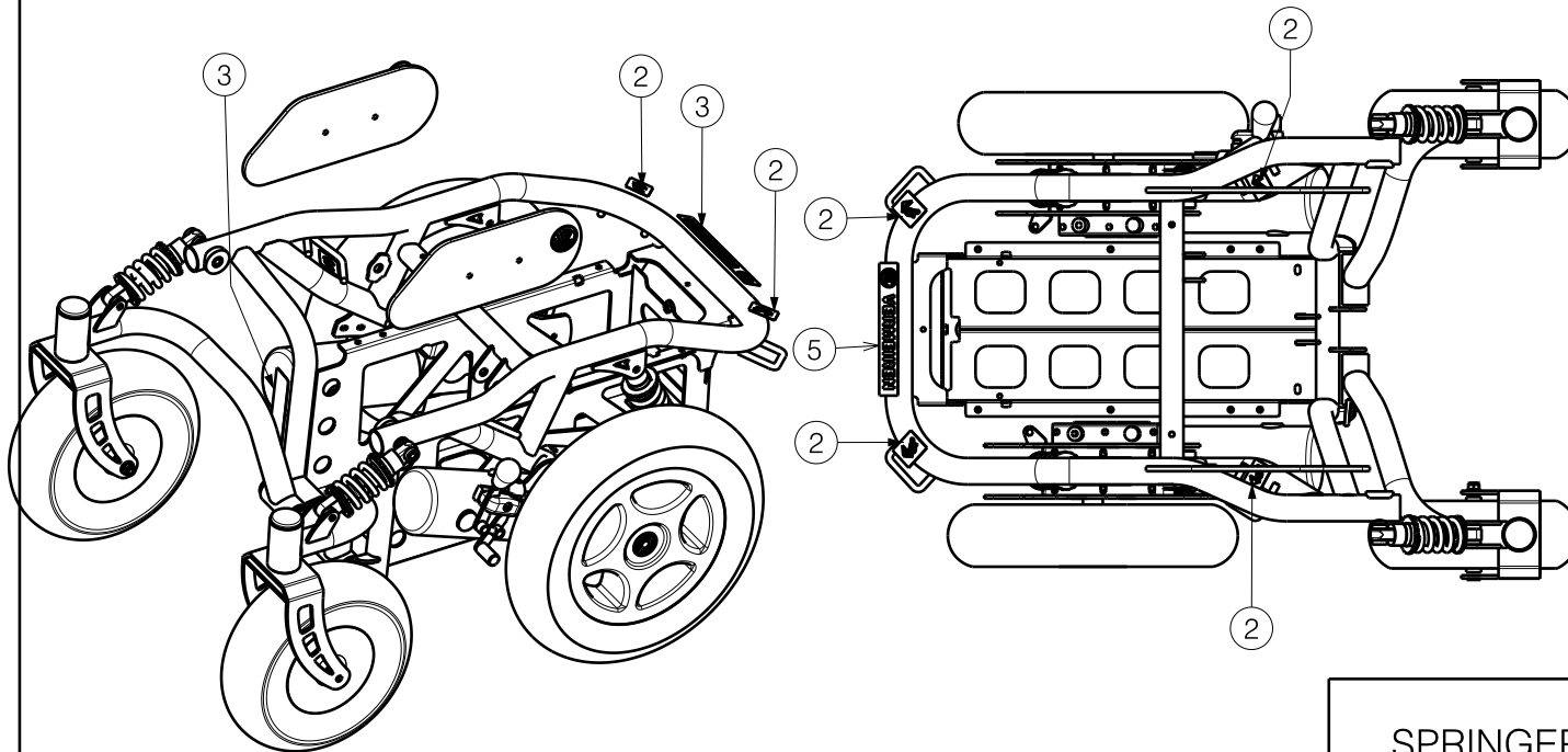
Isometric view Scale: 1:10
